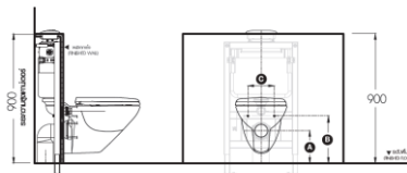
มอดูลซ่อนผนัง สุขภัณฑ์แขวนผนัง แบบกดบน Concealed Tank รุ่น C962172 Top push installation of C962172 concealed tank
